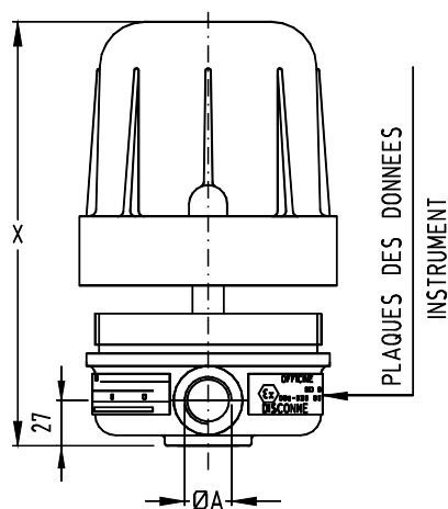
VUE DE COTE BOITIER
