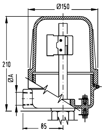
BOITIER POUR GROUPE DECLENCHEMENT SIMPLE
